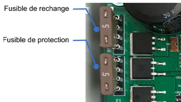
F1 Exemple AN1232
