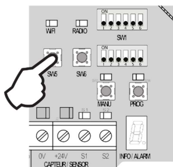
« SW5 » pour fermer la couverture
