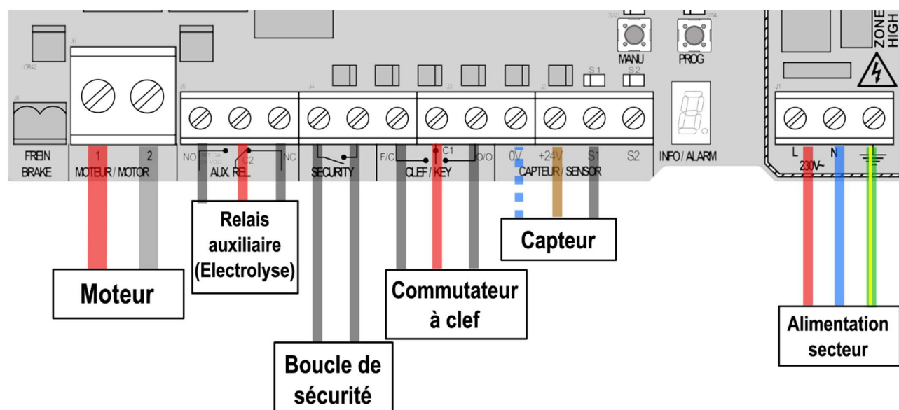
Schéma de câblage coffret AN1232
